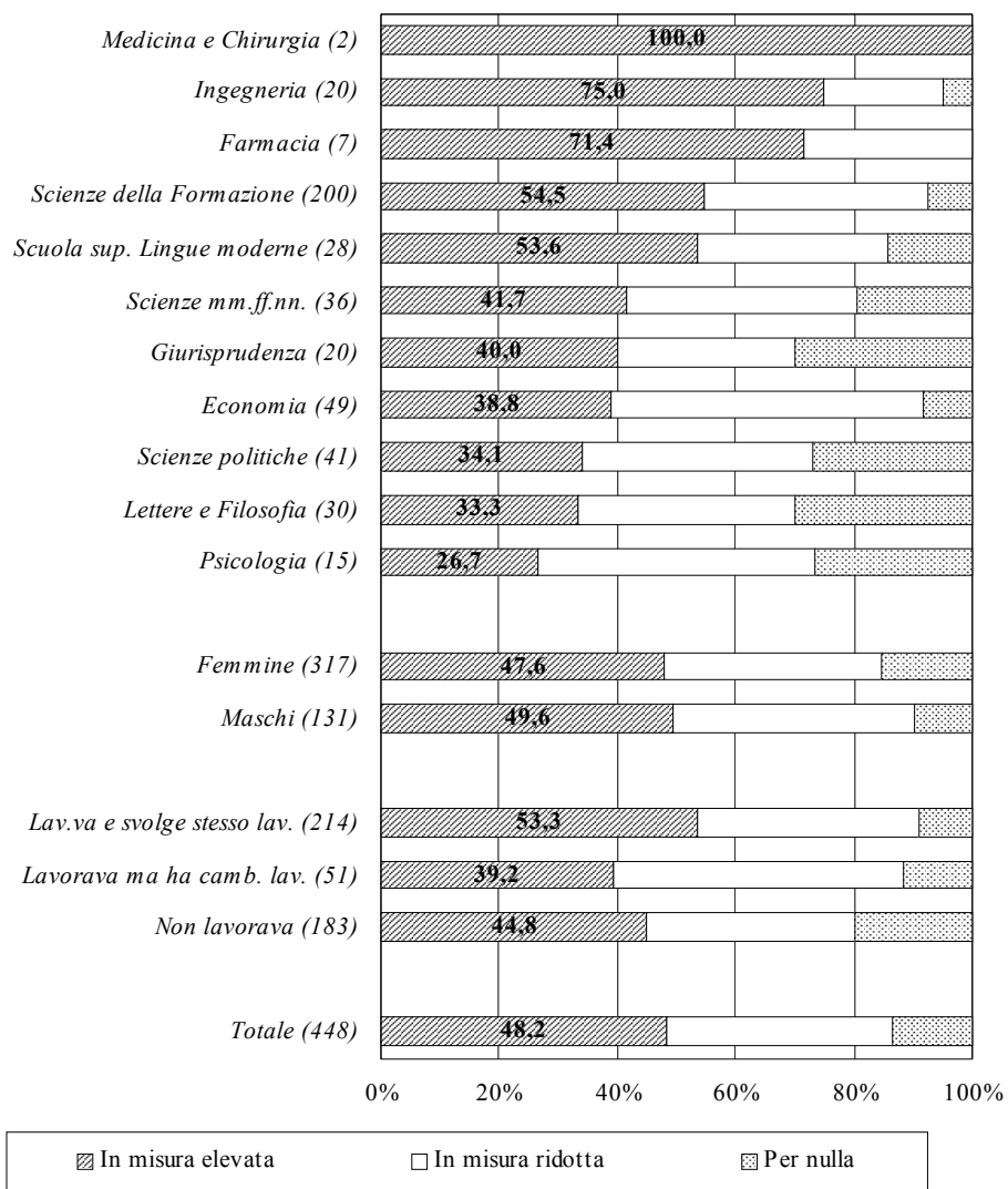
Graf. 4.8 - Occupati: grado di utilizzazione delle competenze acquisite all'università, per facoltà, genere e condizione occupazionale alla laurea (valori percentuali; tra parentesi: numero di intervistati)
