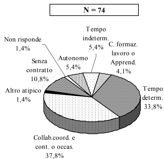
Graf. 5.1 – Laureati non occupati, ma che hanno lavorato dopo la laurea: contratto di lavoro con cui erano stati assunti (valori percentuali)
