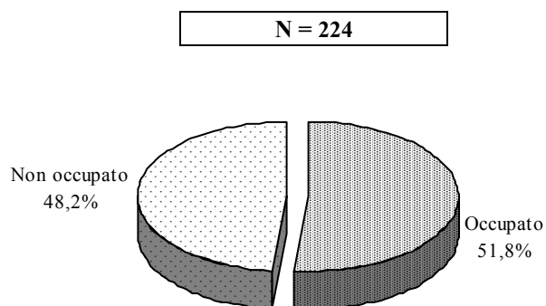
Graf. 6.1 – Laureati in cerca di lavoro: condizione occupazionale ( valori percentuali )
