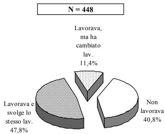
Graf. 4.2 - Occupati: condizione occupazionale al momento della laurea (valori percentuali)
