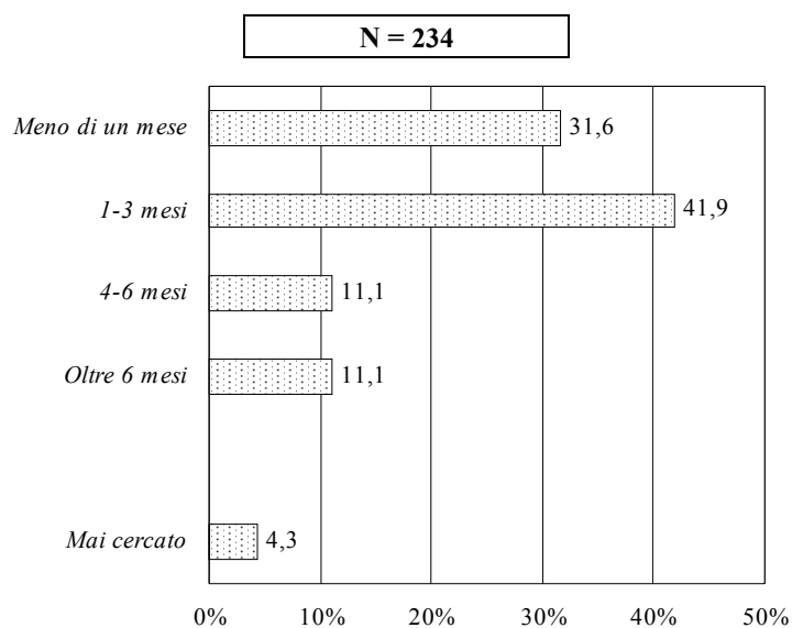
Graf. 4.4 - Occupati che hanno iniziato l'attuale attività dopo la laurea: tempo trascorso tra l'inizio della ricerca di un lavoro ed il suo ottenimento (valori percentuali)
