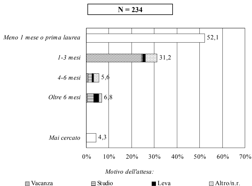
Graf. 4.3 - Occupati che hanno iniziato l'attuale attività dopo la laurea: tempo trascorso tra la laurea e l'inizio della ricerca di un lavoro e motivo dell'attesa prima di iniziare la ricerca (valori percentuali)
