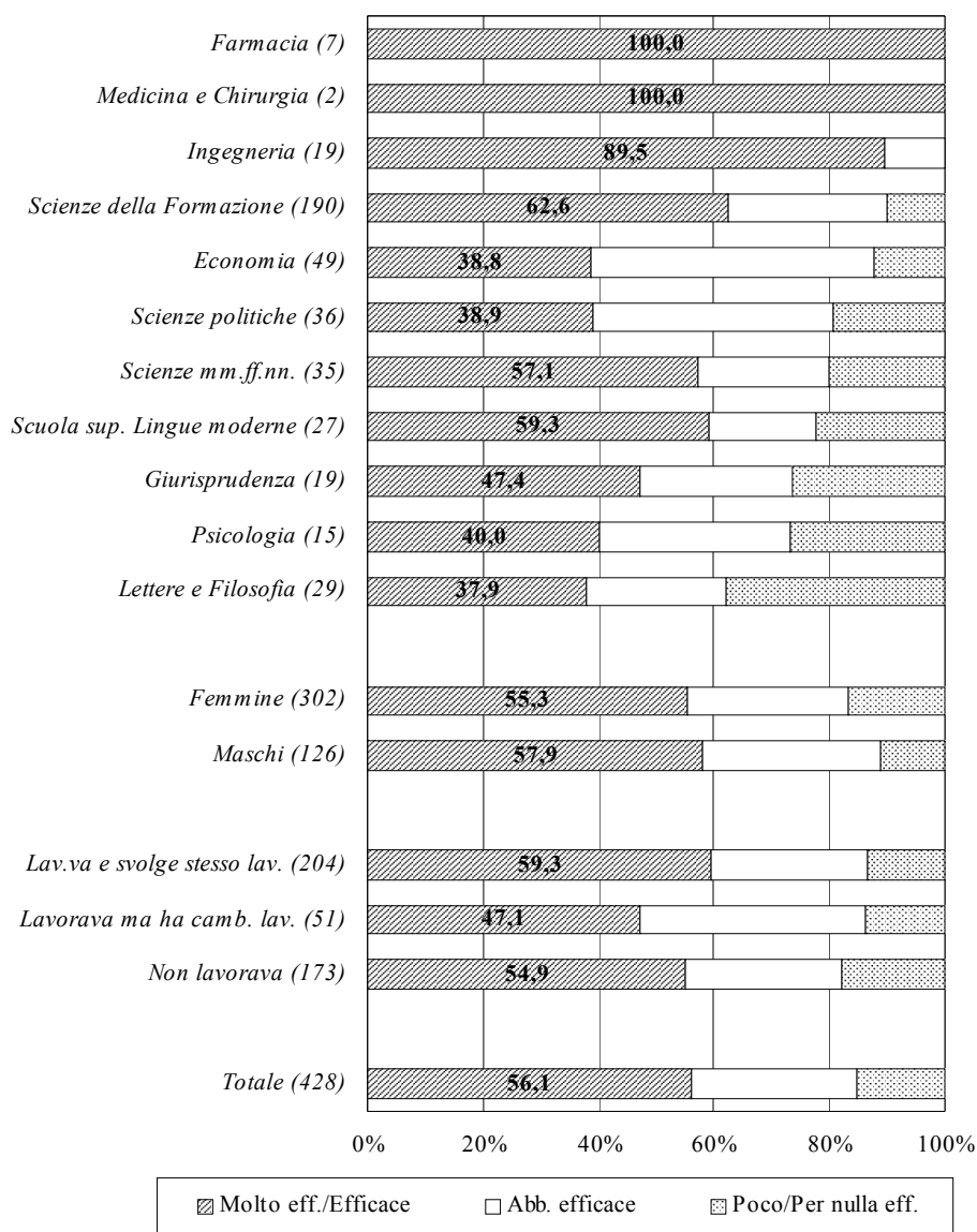
Graf. 4.10 - Occupati: efficacia esterna della laurea, per facoltà, genere e condizione occupazionale alla laurea (valori percentuali; tra parentesi: numero di intervistati che è stato possibile classificare)
