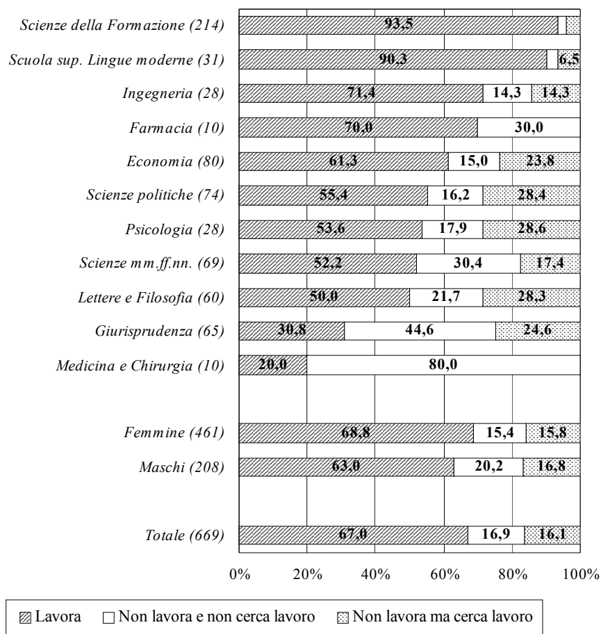
Graf. 3.2 - Condizione occupazionale dei laureati, per facoltà e per genere * (valori percentuali; tra parentesi: numero di intervistati)
