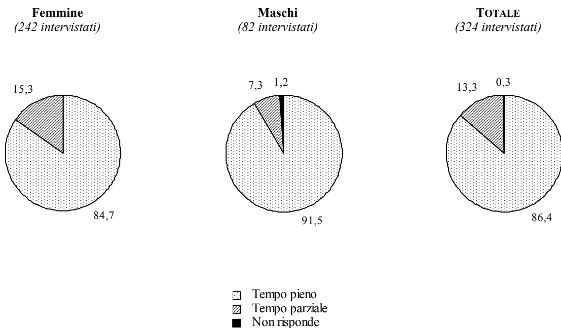
Graf. 4.7 - Occupati alle dipendenze: diffusione del contratto a tempo parziale (part-time), per genere (valori percentuali)
