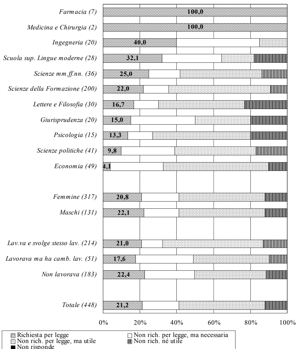
Graf. 4.9 - Occupati: necessità della laurea per l'esercizio dell'attuale lavoro, per facoltà, genere e condizione occupazionale alla laurea (valori percentuali; tra parentesi: numero di intervistati)
